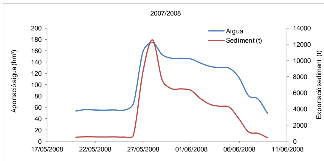
F.8 Hidrograma i sedimentograma del total d'aigua i sediment transferit durant la crecuda de maig de 2008.
