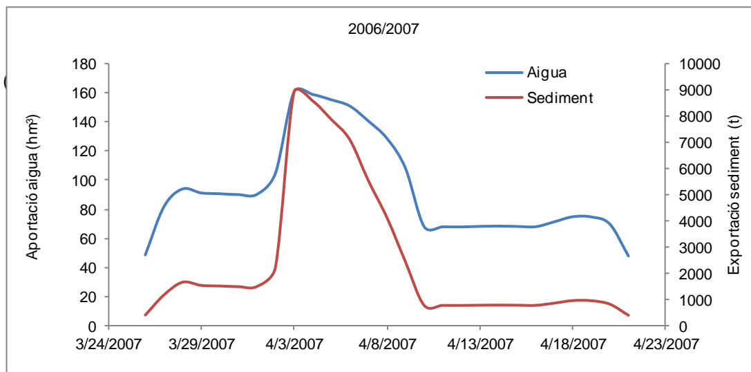
F.7 Hidrograma i sedimentograma del total d'aigua i sediment transferit durant la crecuda del març de 2007.
